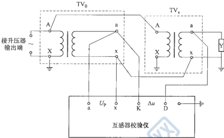
图 A.2 电压互感器检定装置环境电磁场干扰试验接线图
