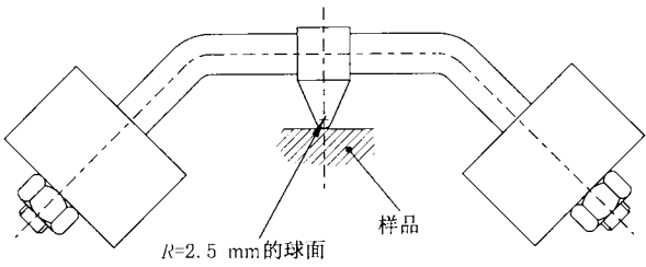
图 10 球压装置
