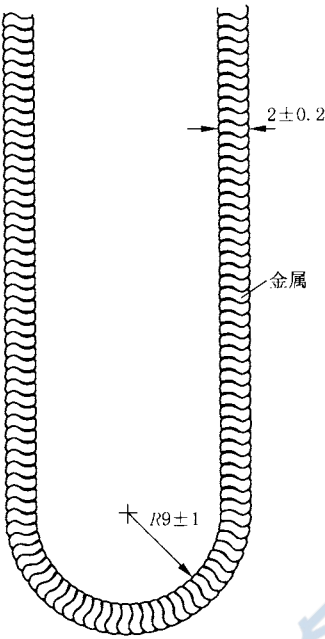
图 29 试验链
