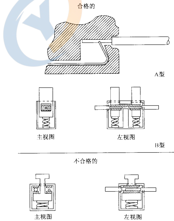
图 17 电气连接件结构图
