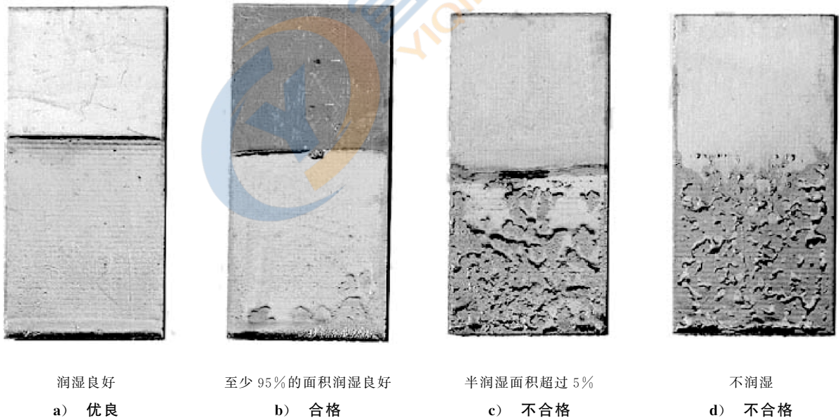
图 12 可焊性评定对照图
