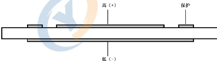
图 37 体积电阻测试连线图
