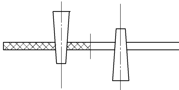
图 33 击穿电压(平行层向)电极插入试样示意图
