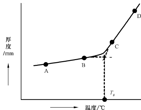
图 18 厚度-温度 TMA 探针法测试曲线图
