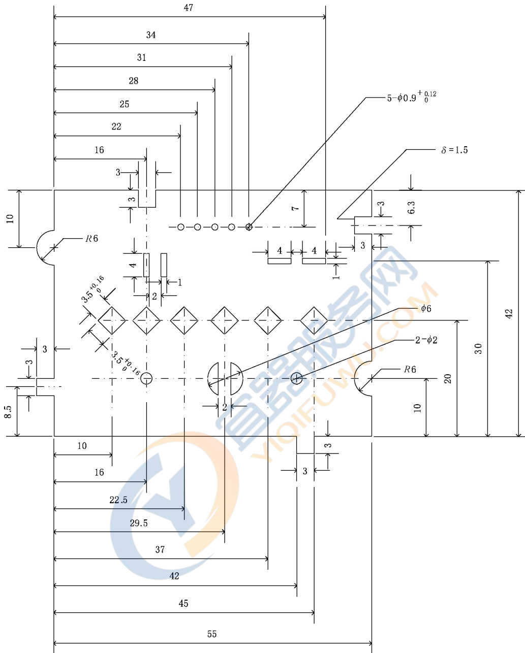
图 31 冲孔性试验冲样图
