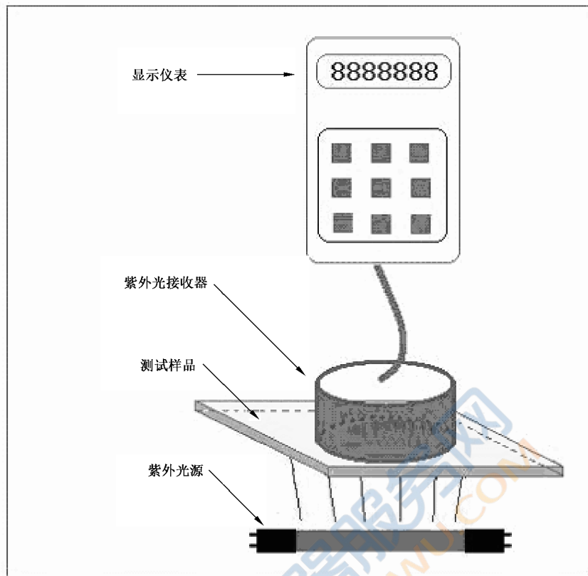
图 22 UV(紫外光)透过率装置示意图
