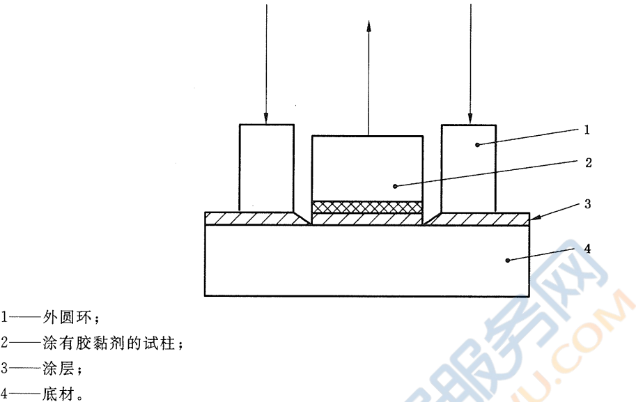
图 5 坚硬底材的试验组合
