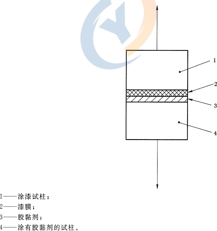
图 6 仅使用试柱的试验组合
