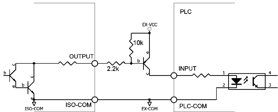
图 10-13 输出到 PLC 正公共端子
