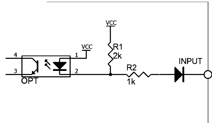
图 10-2 输入端原理图 (Trig)
