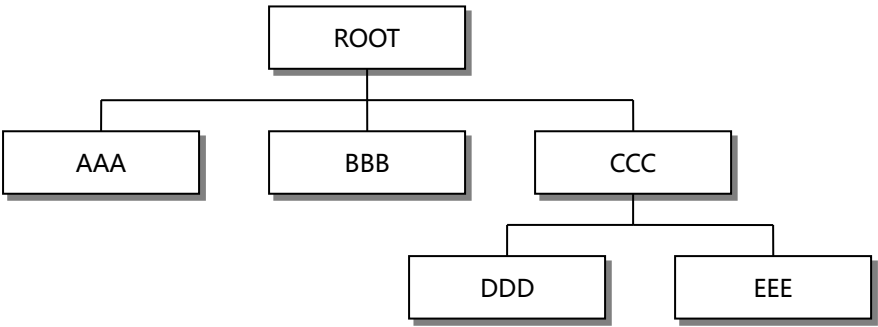
命令树结构
