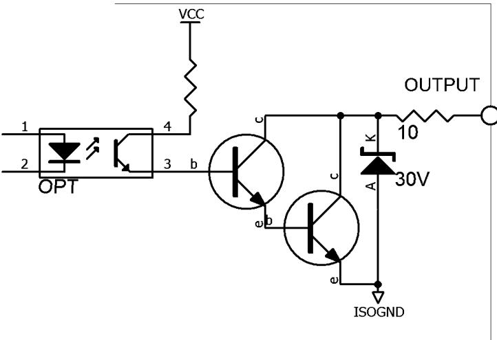
图 10-3 输出端原理图
