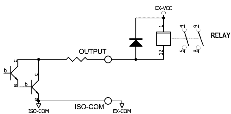
图 10-8 控制继电器
