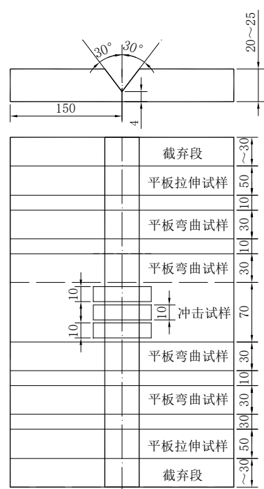
图A. 10 埋弧多道焊对接工艺试件的取样位置
