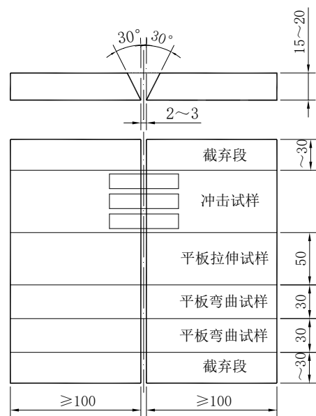
图A. 7 对接焊试件的取样位置
