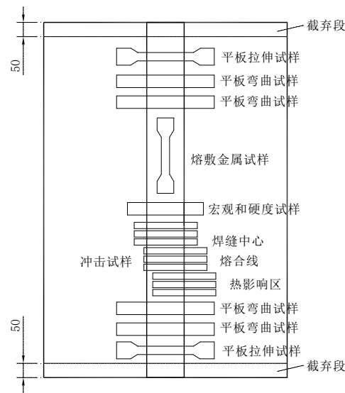
图A.1 平板对接试板的取样位置
