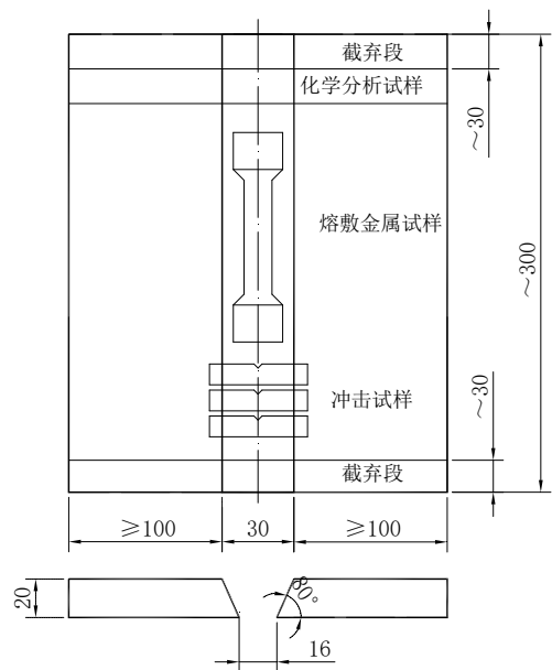
图A. 6 熔敷金属对接焊试件的取样位置
