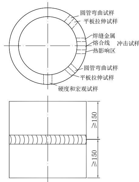
图A.2 管对接试板的取样位置
