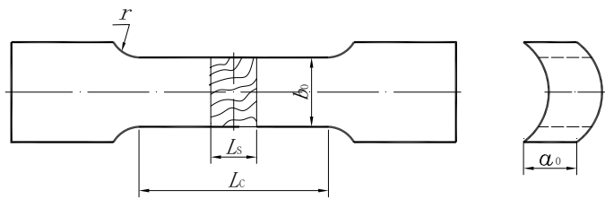
图 23 圆管拉伸试样
