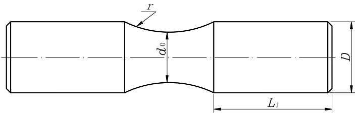
图 7 灰铸铁试样
