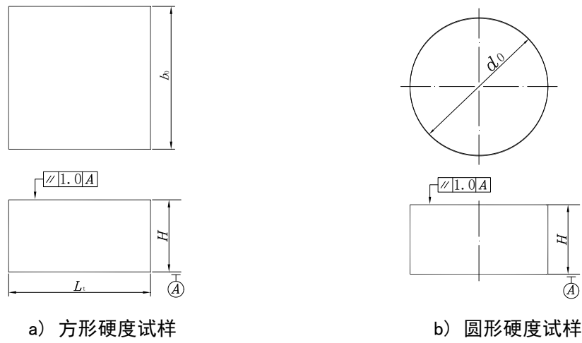
图 9 硬度试样
