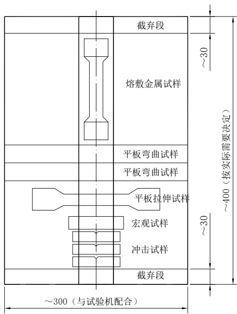
图A. 5 锅炉及受压容器对接焊试件的取样位置
