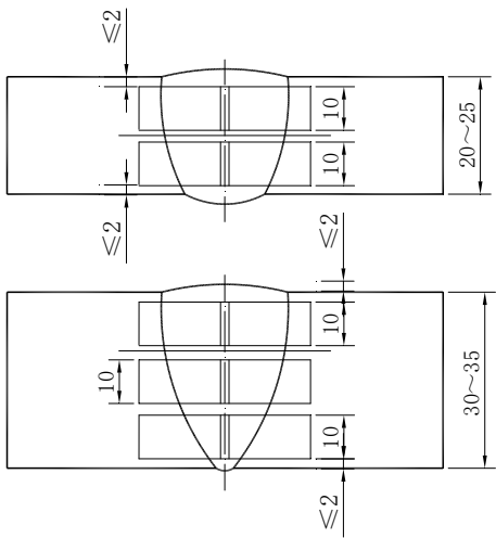
图 A. 13 单面焊接双面成型焊接试件的取样位置
