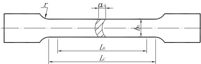
图 5 纵向弧形拉伸试样
