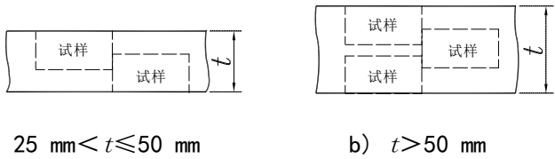
图 22 试件
