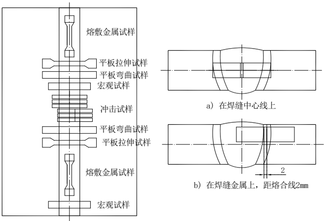
图 A. 12 电渣焊或气电立焊对接焊试件的取样位置
