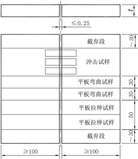
图A. 8 深熔对接焊试件的取样位置
