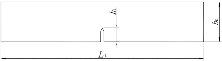
图 13 断口试样
