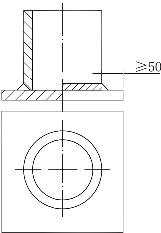
c) 管板角接焊试件的取样位置
