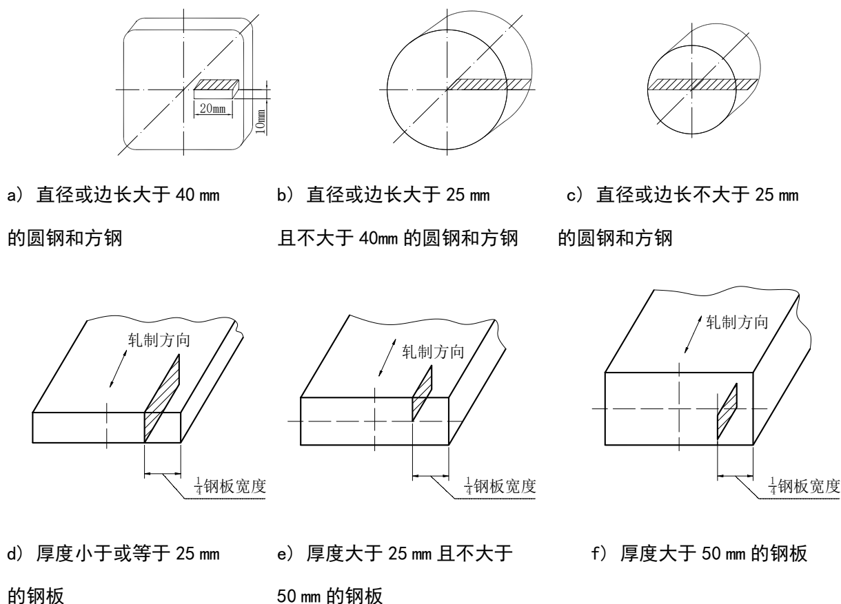
图 14 非金属夹杂物试样取样图
