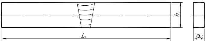
图 28 侧弯试样
