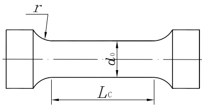
图 4 全厚度试样
