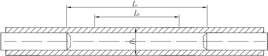
图 6 管段拉伸试样
