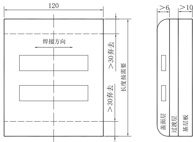
图 18 堆焊焊条试样取样
