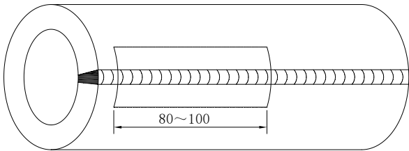
图 15 焊管舟形试样取样
