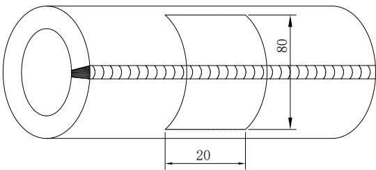
图 16 焊管弧形试样取样
