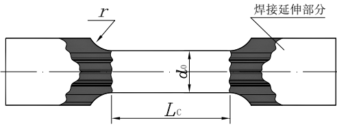
图 3 接长试样
