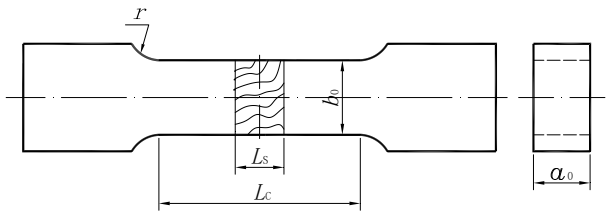
图 21 平板拉伸试样
