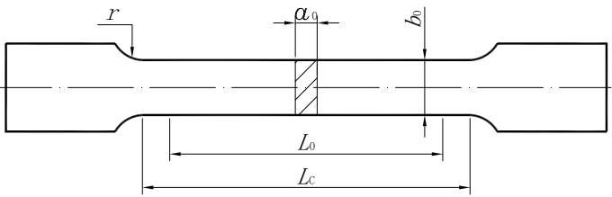
图 2 矩形拉伸试样
