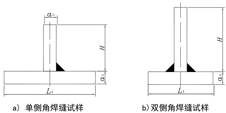
图 30 角焊缝折断试样
