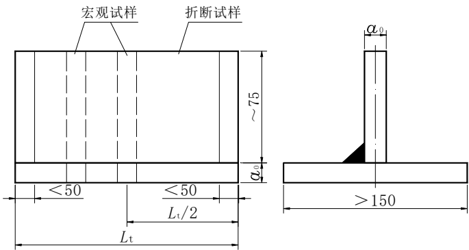
a) 平板角接焊试件的取样位置
