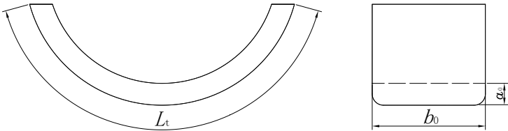
图 11 管材横向弯曲试样
