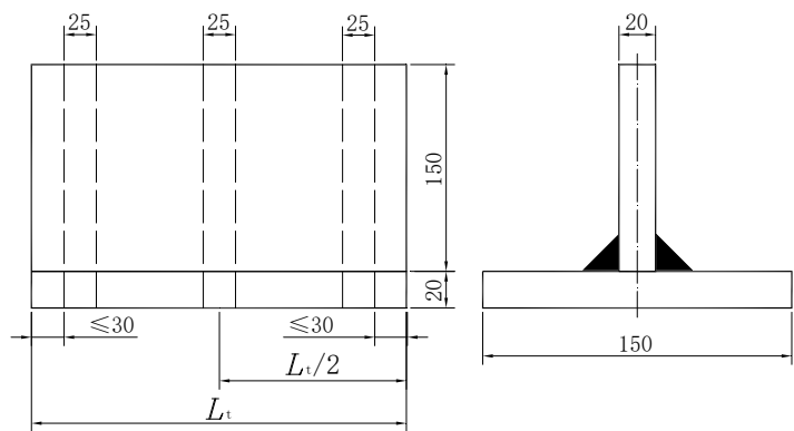
图A. 4 焊条角接焊试件的取样位置
