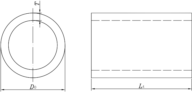
图 12 压扁试样
