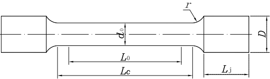
图 1 圆形拉伸试样
