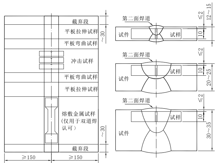
图 A. 11 埋弧双面单道焊工艺试件的取样位置
