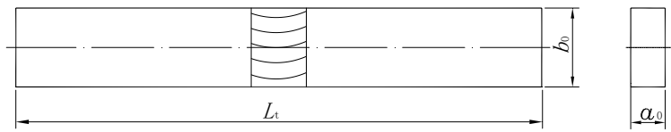
图 26 平板弯曲试样
