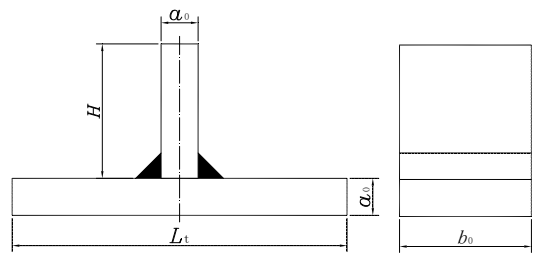
图 29 T 型弯曲试样
