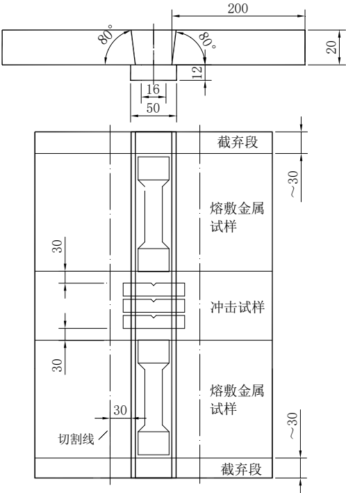
图A. 9 埋弧多道焊熔敷金属试件的取样位置
