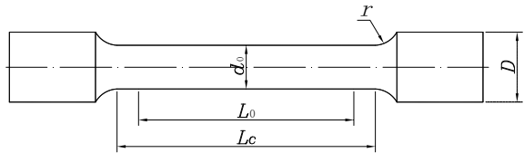
图 24 熔敷金属试样
