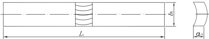
图 27 圆管弯曲试样
