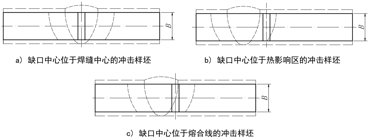
图 25 冲击样坯
