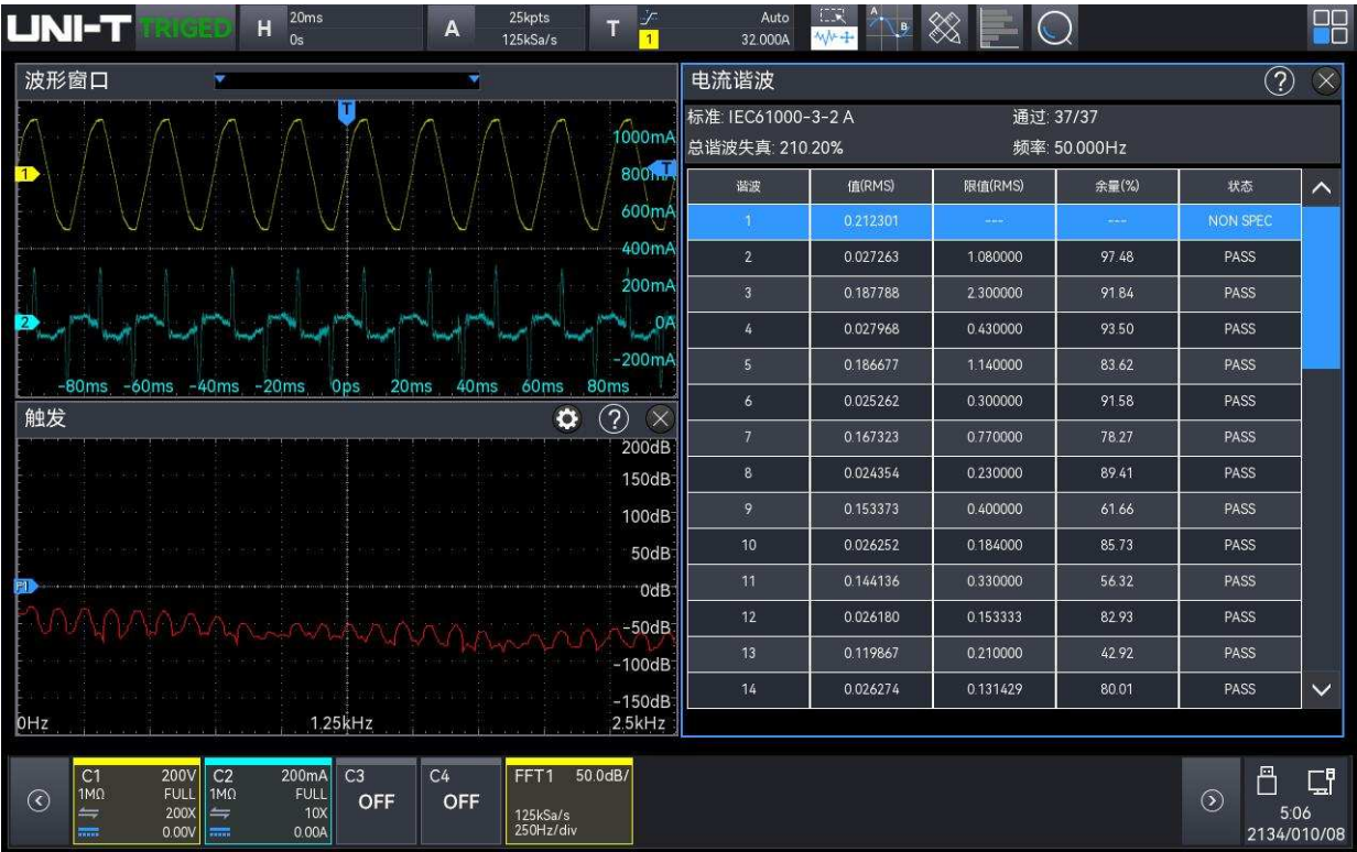
(12) 谐波分析测试结果
