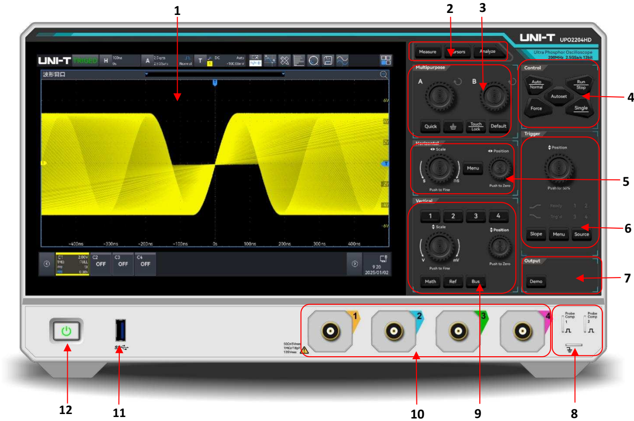
示波器前面板
