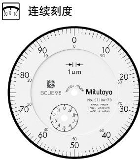
分度值: 0.001 mm 测量范围: 1 mm 2110A-70 防水型 双倍刻度间距型 防震型 宝石轴承型
