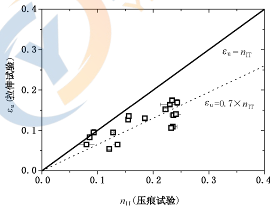
图 A.3 单轴拉伸获得的真应变 \epsilon_u 和压入试验得到的应变硬化指数 n_{IT} 之间的比较
