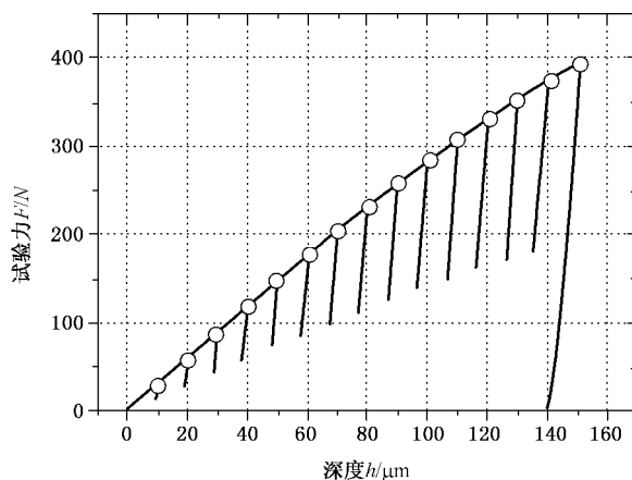
图 5 仪器化压入试验得到的压入试验力-深度曲线
