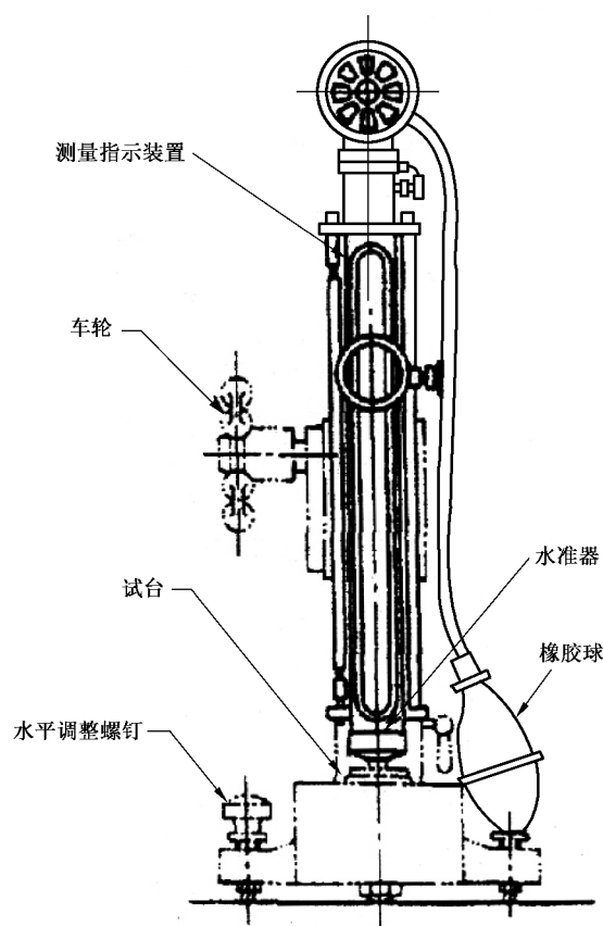
图 A.2 C 型(目测型)硬度计示意图
