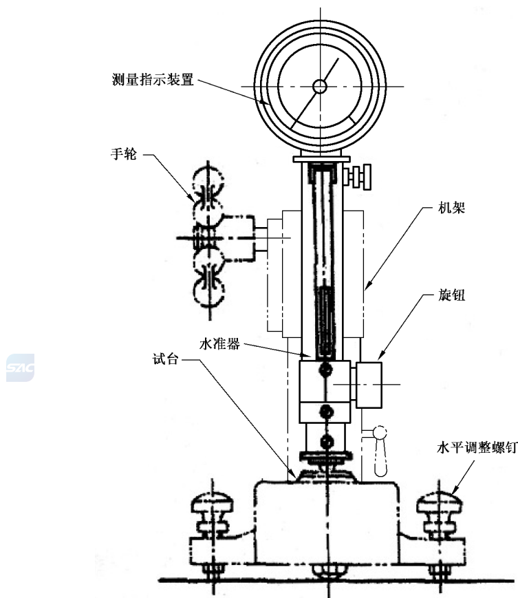
图 A.1 D 型(指示型)硬度计示意图
