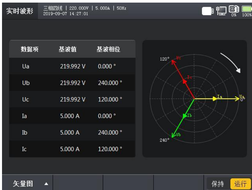
图 7-6 实时波形-相量图
