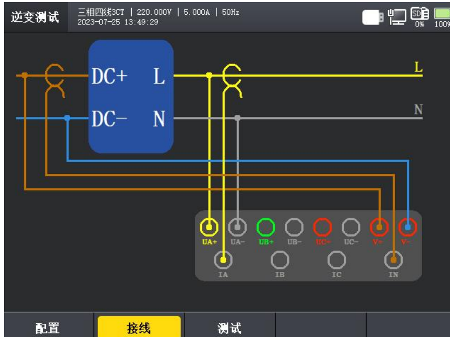
图 9-3 逆变测试-单相逆变器接线
