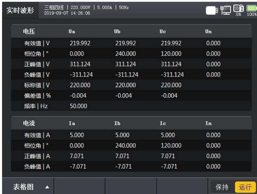
图 7-5 实时波形-表格图 3
