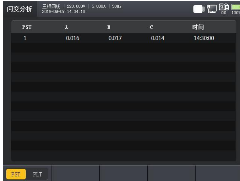
图 7-15 闪变分析
