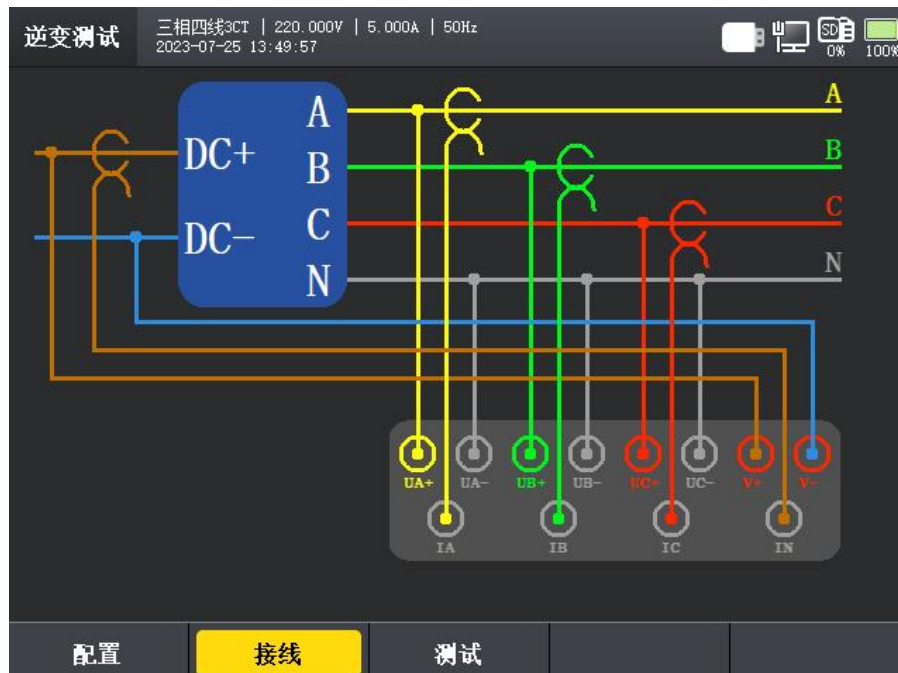
图 9-4 逆变测试三相逆变器接线
