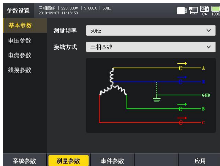
图 5-5 测量参数-基本设置
