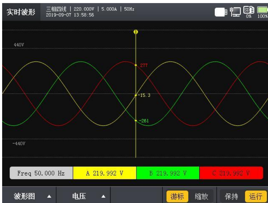
图 7-2 实时波形
