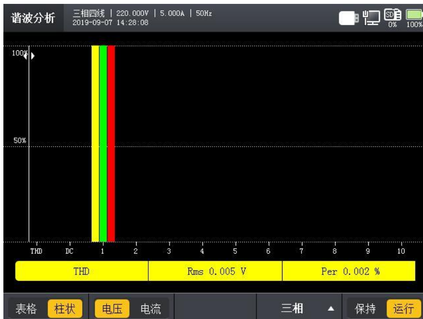
图 7-8 谐波分析-柱状图
