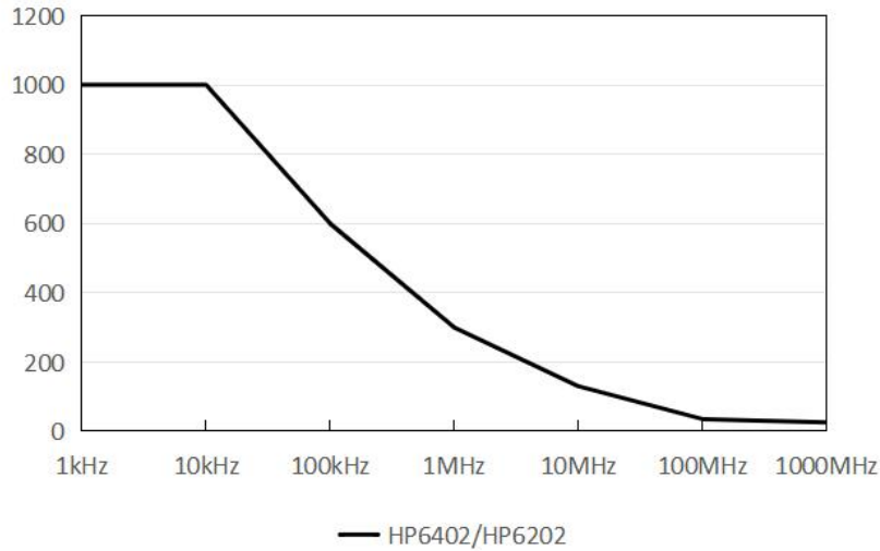
最大有效值 (Vrms) VS 频率曲线
