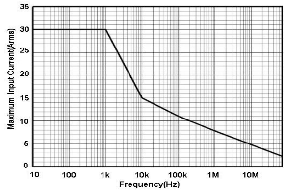
图 2.b HCPR8030C 最大测量电流 VS 频率曲线
