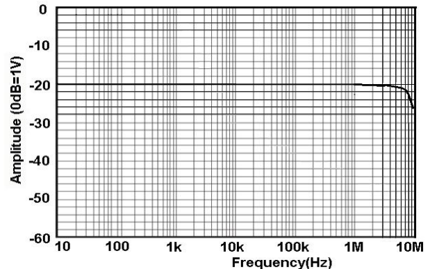
图 13.b HCPR8300A 幅频曲线
