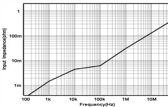
图 3.a HCPR8030 输入阻抗 VS 频率曲线
