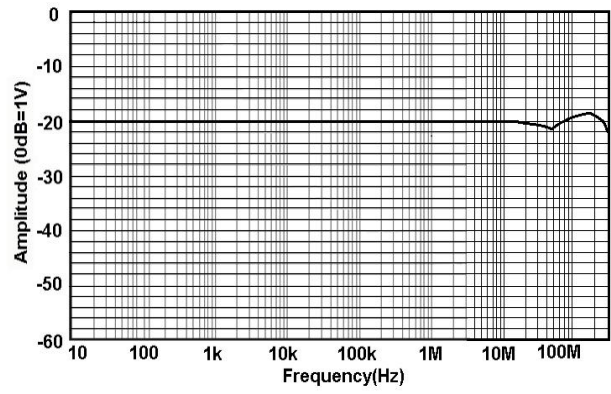
图 1.d HCPR8030H 幅频曲线
