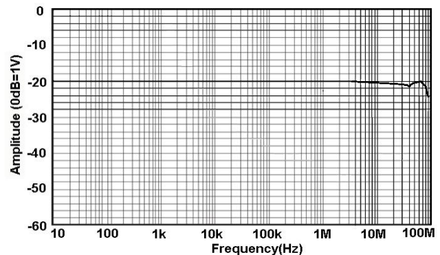
图 1 .b HCPR8030C 幅频曲线
