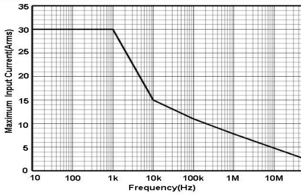
图 2.a HCPR8030 最大测量电流 VS 频率曲线
