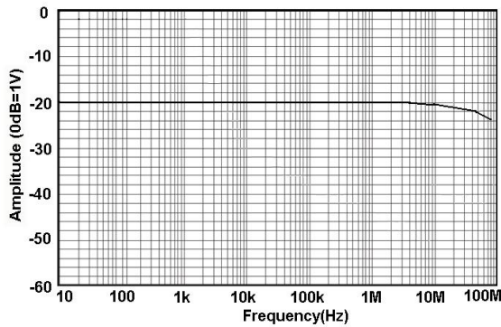
图 4 HCPR8050 幅频曲线
