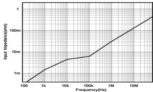
图 3.b HCPR8030C 输入阻抗 VS 频率曲线
