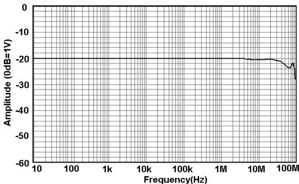
图 1 .a HCPR8030 幅频曲线
