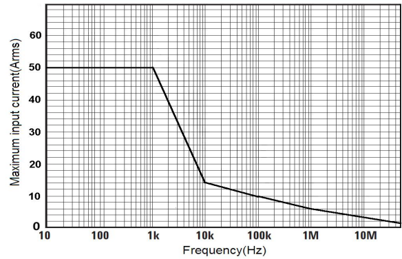
图 5 HCPR8050 最大测量电流 VS 频率曲线 (超过该曲线所示最大电流连续使用会导致探头烧毁)
